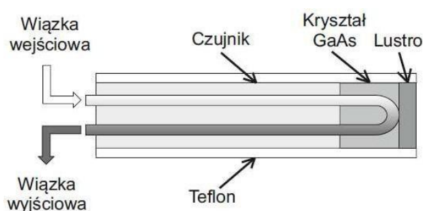
Rysunek 1. Schemat działania czujnika opartego na technologii arsenku galu. Źródło: www.fiso.com
