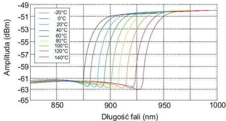
Rysunek 2. Widmo czujnika GaAs mierzone optycznym analizatorem widma dla temperatur od -20\text{ }^{\circ}\text{C} do +140\text{ }^{\circ}\text{C} z różnicą co 20\text{ }^{\circ}\text{C} .
