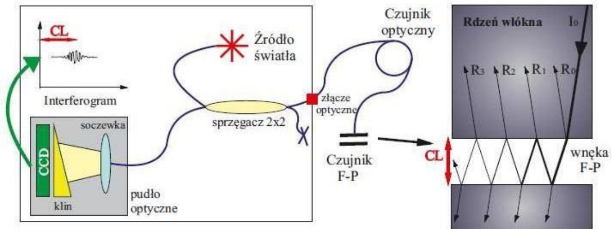
Rysunek 3. Schematyczny opis bezwzględny sygnału pomiarowego F-P opartego na interferencji światła białego (po lewej) i struktura interferometru pomiarowego F-P pokazująca bieg promieni uzyskanych przez rozchodzenie się wiązki światła w rdzeniu włókna optycznego (po prawej).
